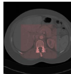
Cropping
